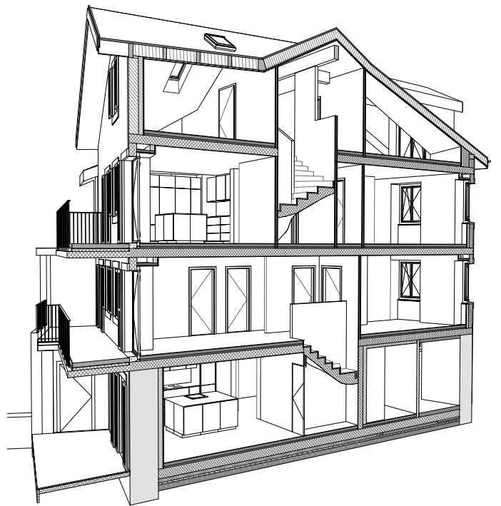
COUPE 3D
